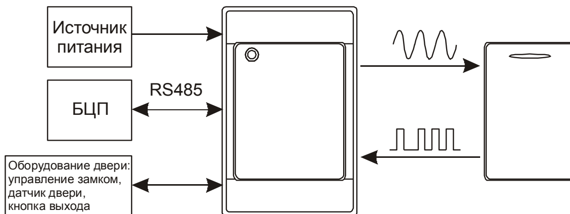
Рис. 1 Функциональная схема работы УСК
