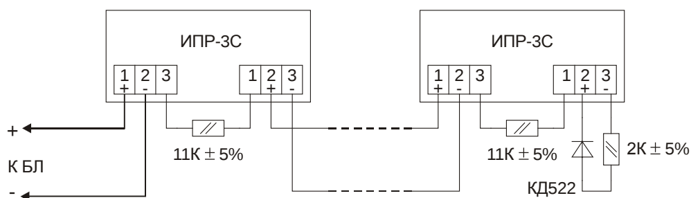
Рис. 23 Схема включения ИПР-ЗС
