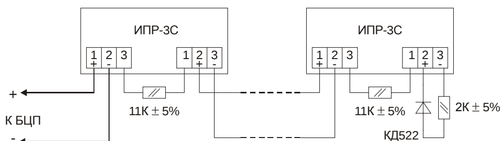
Рис. 27 Схема включения ИПР-3С
